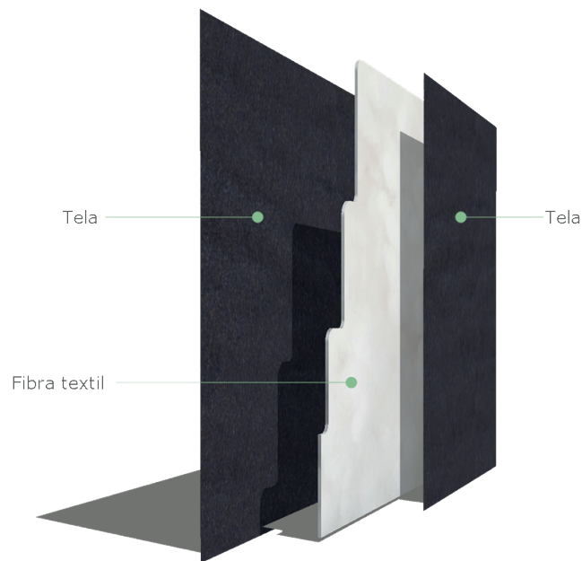
Detalle 1. Isométrico de Blanket Residential absorbente.
