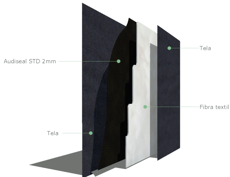
Detalle 2. Isométrico de Blanket Residential aislante.
